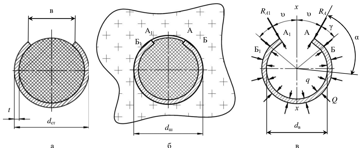
Рис. 4. Поперечное сечение, выполненное в передней части стержня: а – сечение стержня анкера до установки в шпур; б – сечение после установки в шпур; в – схема нагружения стержня анкера
